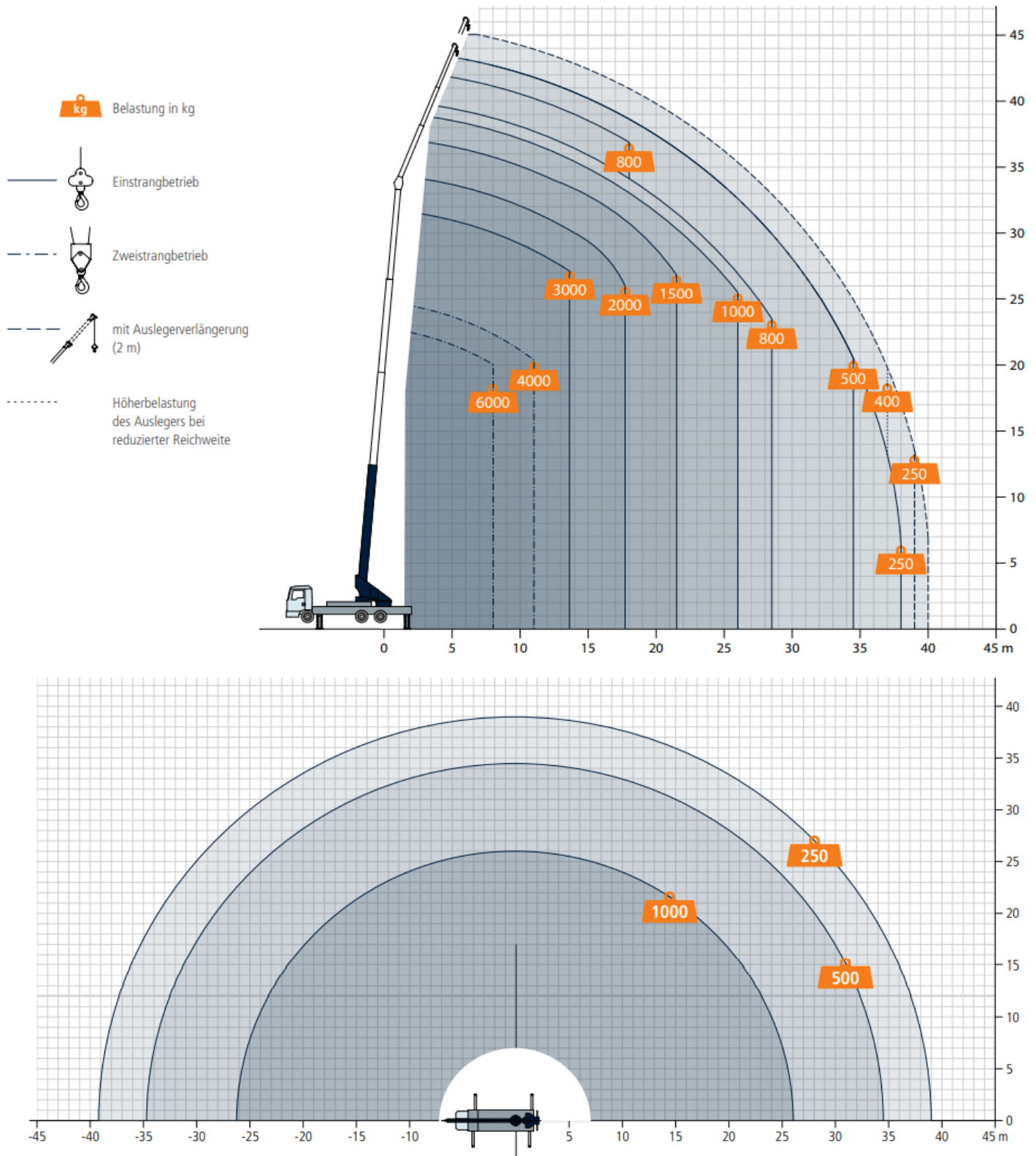
Abbildung 1: Lastdiagramm Autokran (Quelle: www.boecker.de/autokrane )
