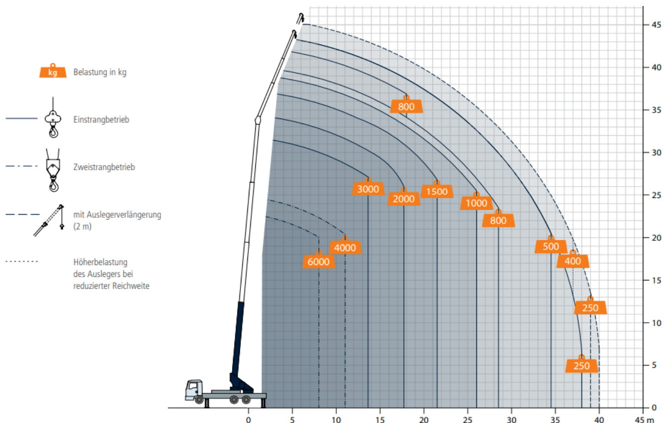
Abbildung 1: Lastdiagramm Autokran (Quelle: www.boecker.de/autokrane )
